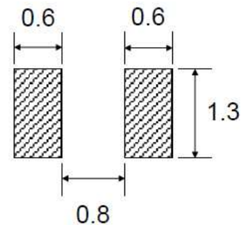
ランドパターン / Land pattern
